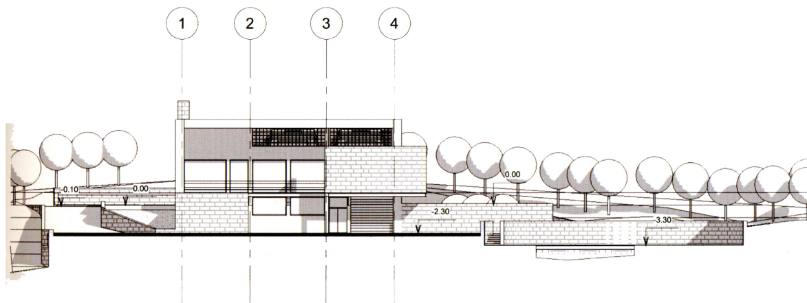
13 Longitudinal profile A101 1 : 200
